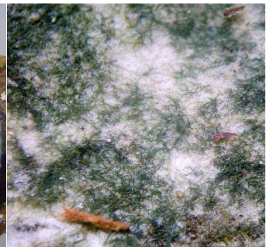
12 Dictyonema HYGROPHORACEAE
